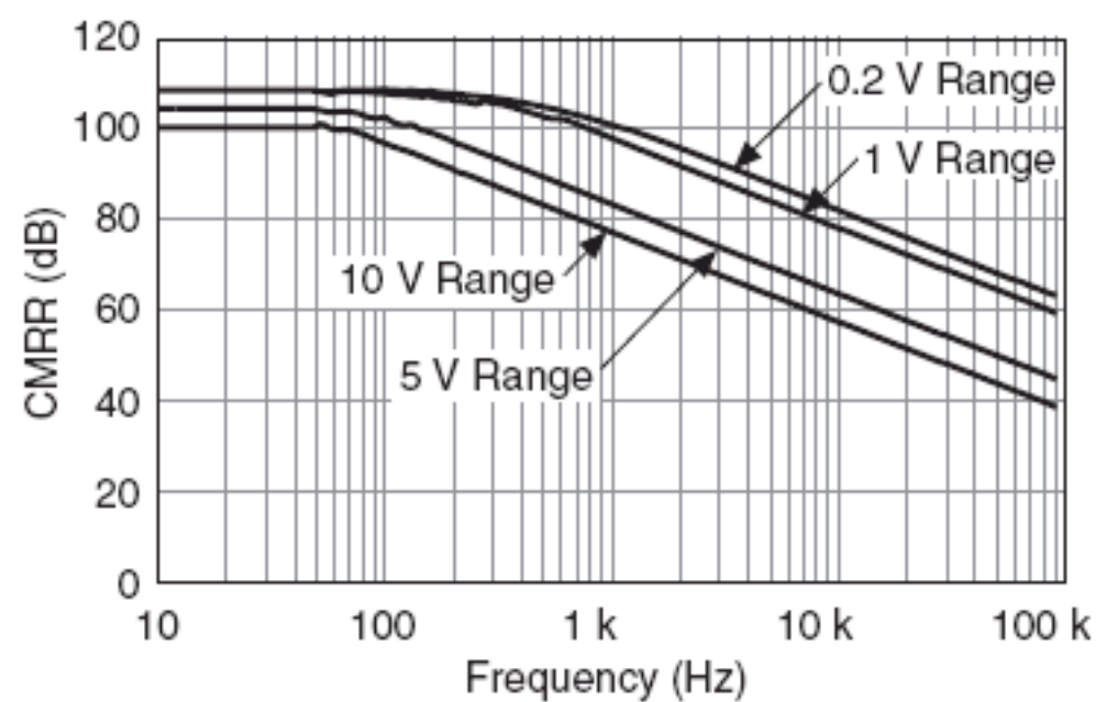
AI <0..79> CMRR
